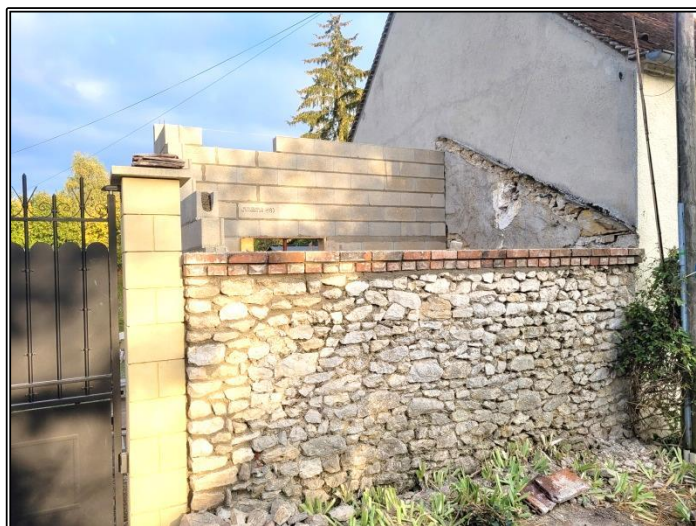
Suite élévation du mur côté cour et côté rue
